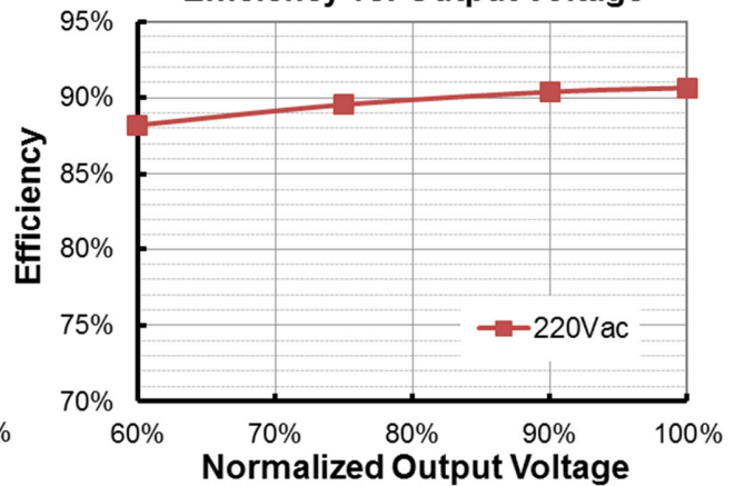
EBS-040S070BT2 (I o =700mA)
