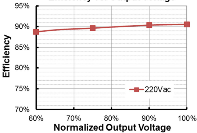
EBS-040S070BT2 (I o =450mA)
